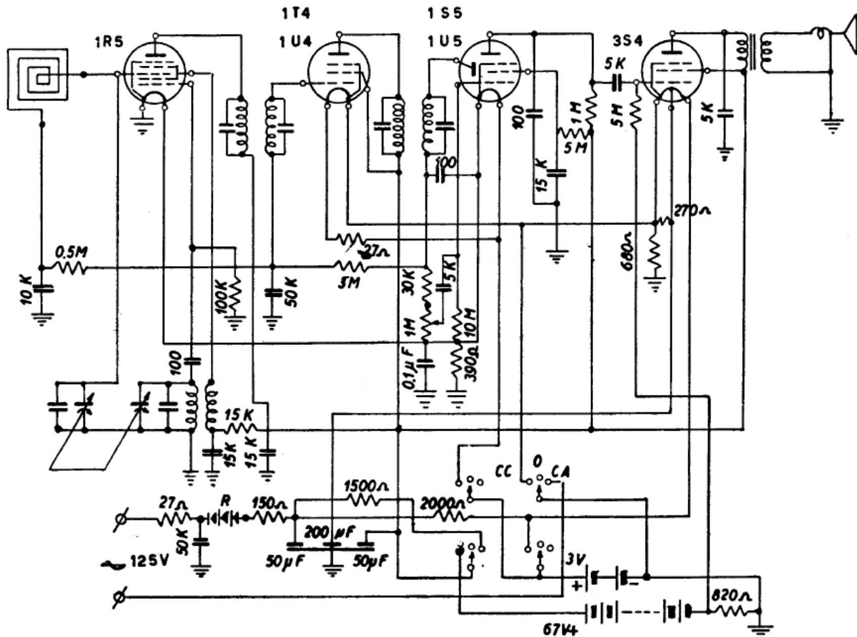
SINTOMAGIC RADIO (REOM) - Mod. B3. Apparecchio portatile a pile-rete di tipo a tre vie (B-CC-CA). Gamma onde medie, sintonia a condensatore variabile. Media frequenza 470 kc/s. Rettificatore a selenio.
